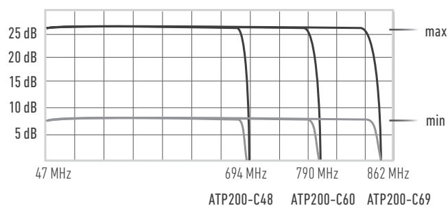
Gráficas de regulación de ganancia
